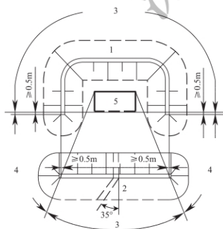
图 5.4.1-1 标准防护土堤的平面防护范围
