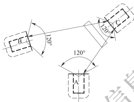
图 5.3.5-5 覆土库方位关系图:1. 每个仓库均为前面到前面 2. C 为前面有防护屏障, A 和 B 为前面无防护屏障
