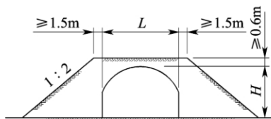
图 8.9.4 覆土库的覆土剖面示意图
